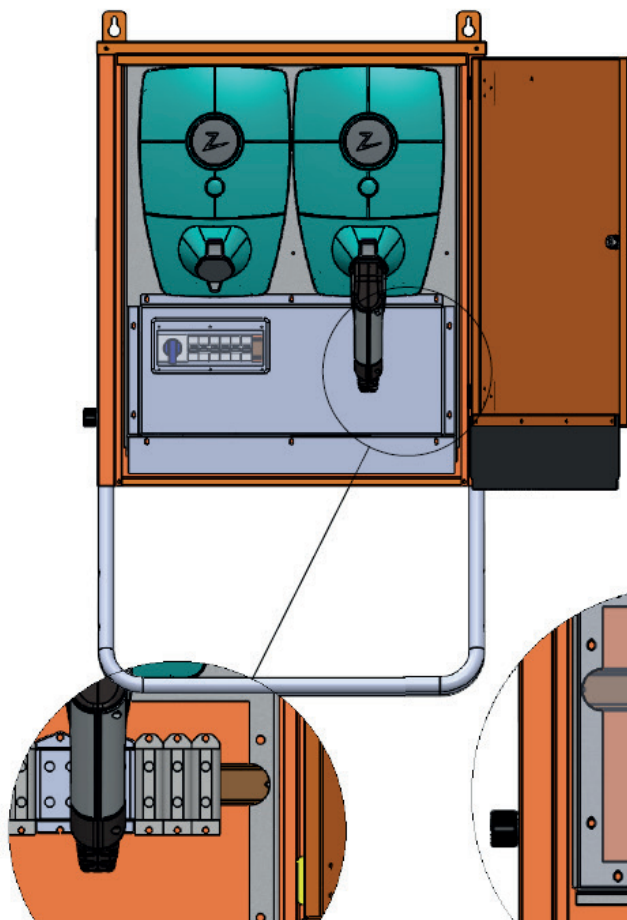
ARTIKEL S9502-01 LCF125.Z20
